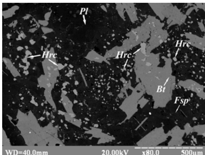
Рис. 3. Морфологические особенности герцинита в ксенолите биотит-полевошпатового кристаллосланца Малинского участка. Изображение под электронным микроскопом. Условные обозначения соответствуют приведенным на рисунке 2
