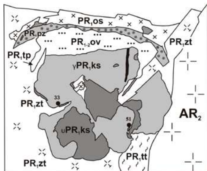
Рис. 1. Схема геологического строения Коростенского плутона. Условные обозначения: PR,ks – граниты, анортозиты и габброиды коростенского комплекса; PR,zt – граниты и мигматиты житомирского комплекса; PR,os – граниты, гранодиориты и диориты осницкого комплекса; PR,pz – граниты и метасоматиты пержанского комплекса; PR,tt – гнейсы и кристаллосланцы тетеревской серии; PR,tp – вулканогенно-теригенные образования топильнянской серии; PR,ov – вулканогенно-теригенные образования овруцкой серии. Точки отбора образцов герцинитсодержащих ксенолитов: 33 – Пугачевский участок, 51 – Малинский участок
