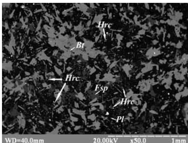
Рис. 2. Характер распределения герцинита в ксенолите биотит-полевошпатового кристаллосланца Пугачевского участка. Изображение под электронным микроскопом. Условные обозначения: Hrc – герцинит, Bt – биотит, Fsp – калиевый полевой шпат, Pl – плагиоклаз
