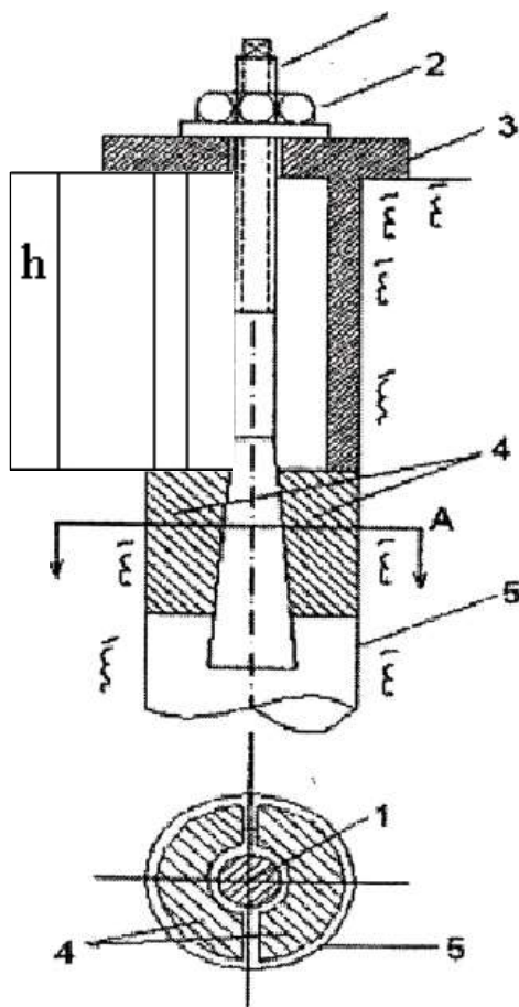
Рисунок 1. Пристрій для утворення направлених тріщин у шпурах
