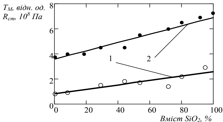
Рисунок 2. Залежність межі міцності при одновісному стисканні – R ст (1) і твердості за шкалою Мооса – T М (2) від вмісту оксиду кремнію (SiO 2 )
