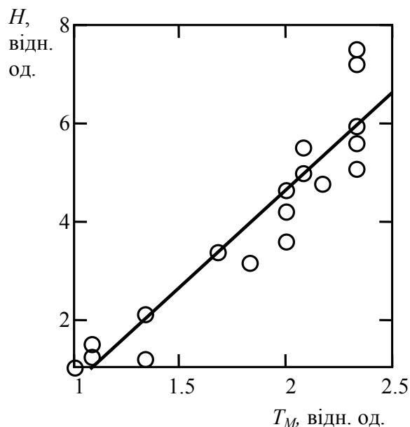
Рисунок 2. Залежність мікротвердості ( H ) та твердості за шкалою Мооса ( T_M ) у відносних одиницях
