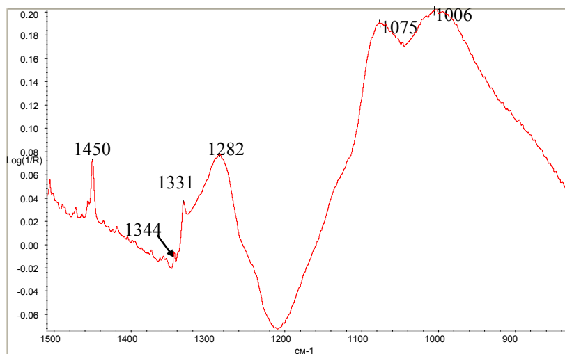
Рисунок 7. Облагороджені алмази змішаного типу Ib+IaA (пік 1282\text{ см}^{-1} , 1344\text{ см}^{-1} ) фіолетового кольору
