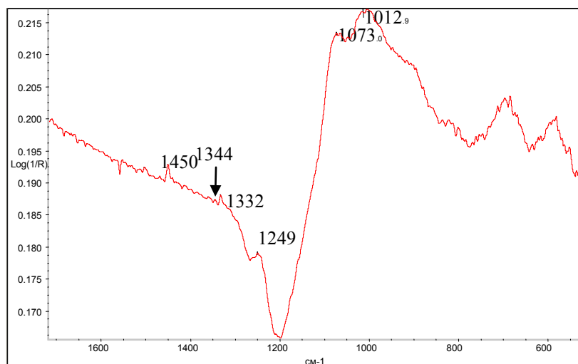
Рисунок 6. Облагороджені алмази типу Ib (пік 1344\text{ см}^{-1} ) фіолетового кольору
