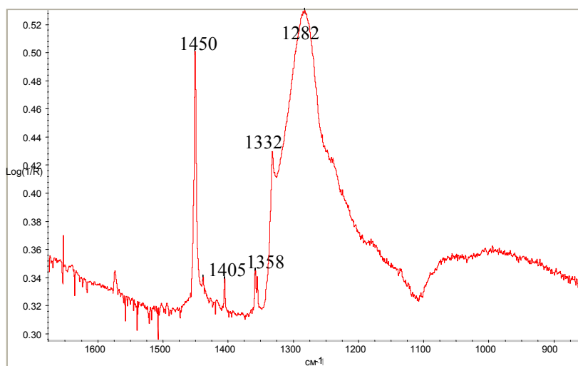
Рисунок 4. Облагороджені алмази типу IaA (пік 1282 \text{cm}^{-1} ) жовто-оранжевого кольору
