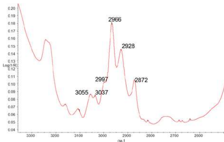
Рисунок 6. Спектр синтетичної смоли в природному смарагді
