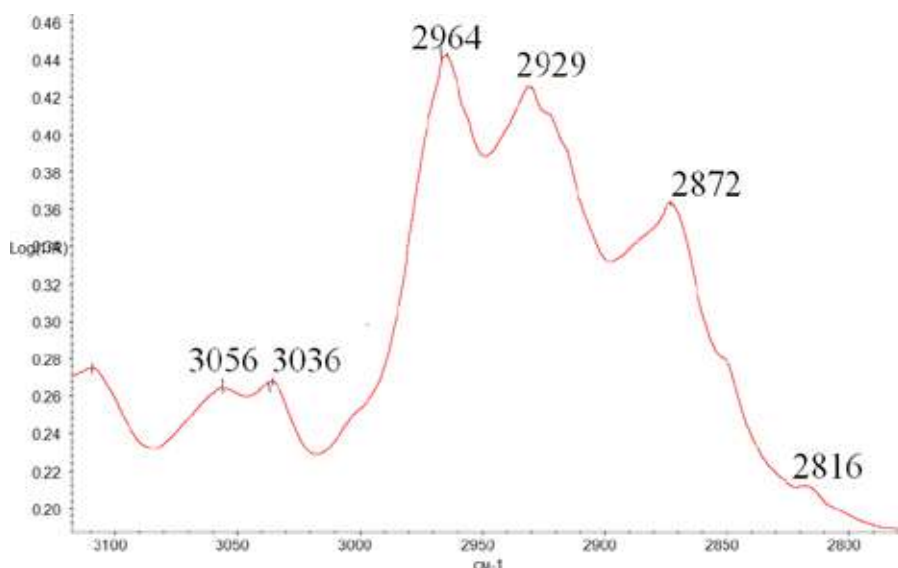
Рисунок 7. Спектр синтетичної смоли в природному смарагді
