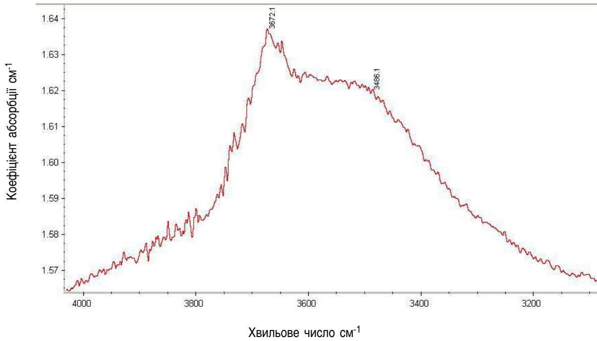
Рисунок 9. Пік близько 1650 \text{cm}^{-1} у природному благородному опалі (Австралія)
