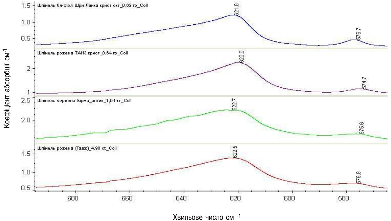
Рисунок 5. Пік близько 625 \text{ cm}^{-1} у шпінелі блідо-фіолетовій (Шрі-Ланка), рожевій (Танзанія), червоній (Бірма), рожевій (Таджикистан)
